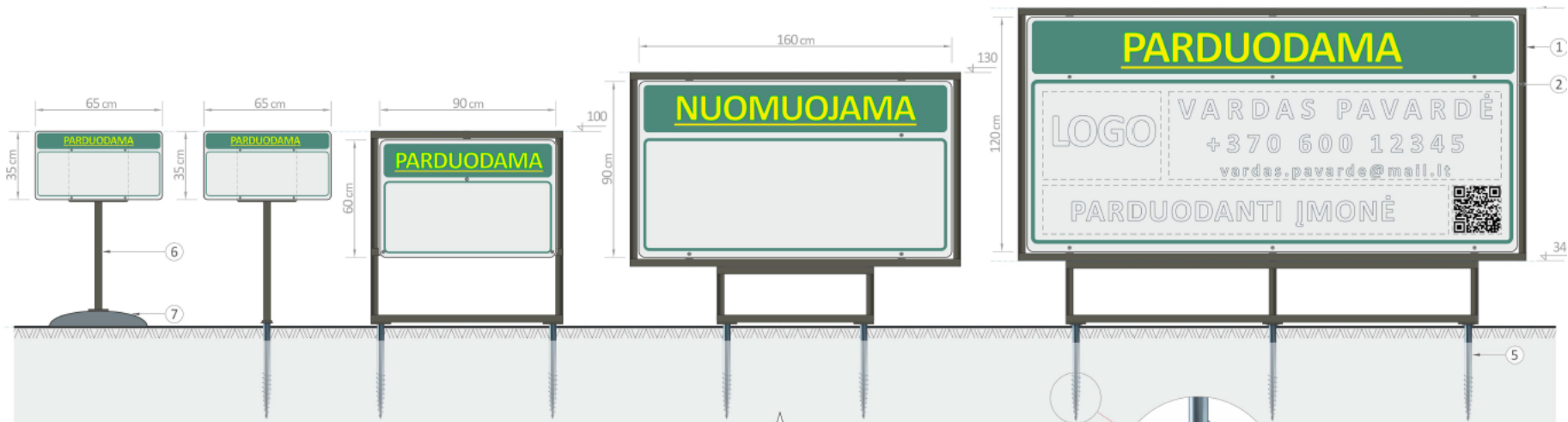
TIPAS Nr. NK.L 2** plotas -0,45 m 2
